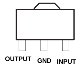
SOT-89 78L12CPK
