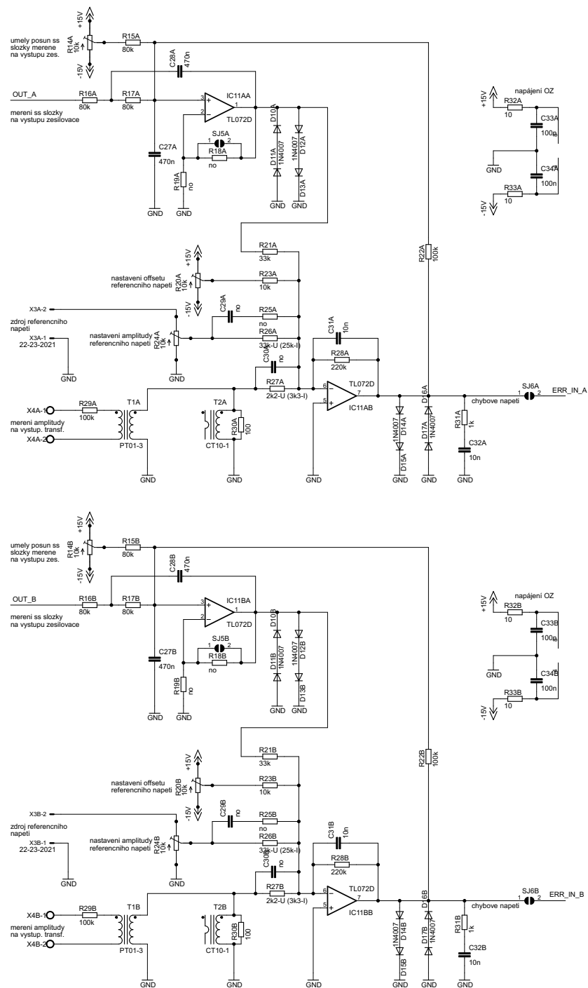
Obrázek 42: Schéma zapojení - list 3
