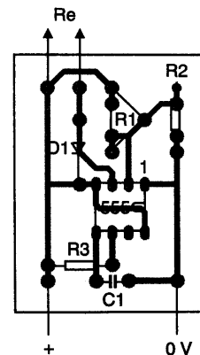
Obr. 75. Deska s plošnými spoji C336 zapojení z obr. 73 pro všechny druhy senzorového obvodu a desky, osazené součástkami ( R_2 je podle potřeby buď fotorezistor nebo termistor)
