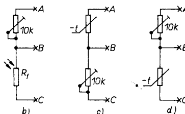
Obr. 3. Poplachové zařízení, základní zapojení, aktivace zatemněním fotorezistoru a), aktivace osvětlením b), poklesem teploty c), zvýšením teploty d)
