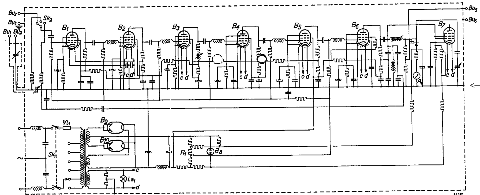
Fig. 5 Principeschema
