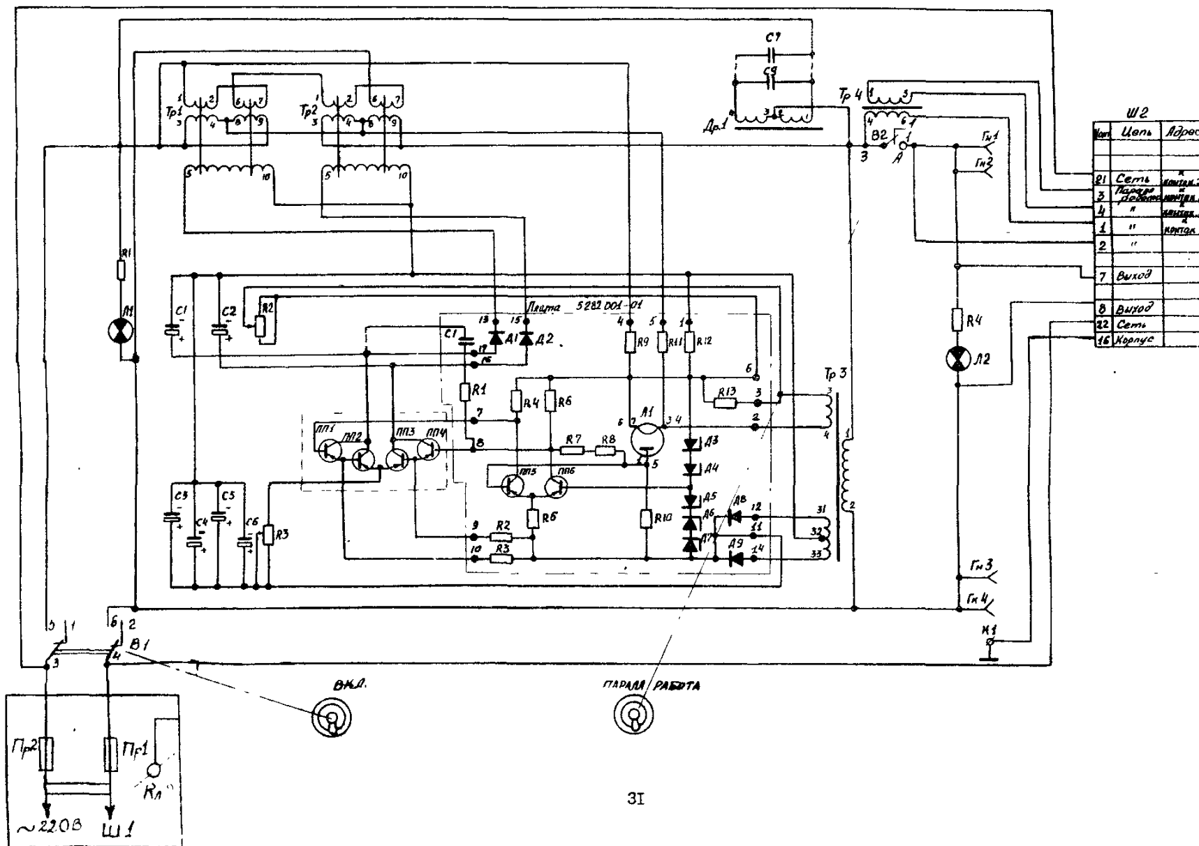
Схема электрическая принципиальная стабилизаторов напряжения сети БЭ-2 /БЭ-3/
