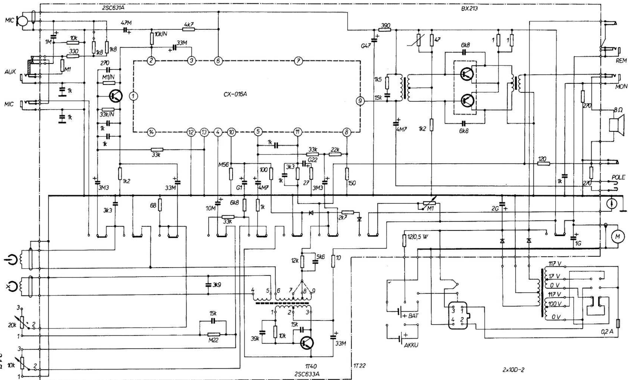
Obr. 168. Schéma zapojení magnetofonu SONY TC-95
