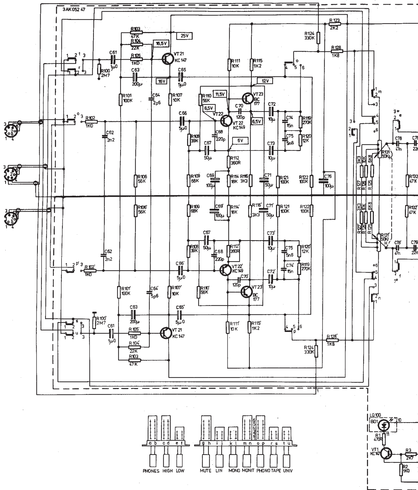
Obr. 2. Schéma zapojení
