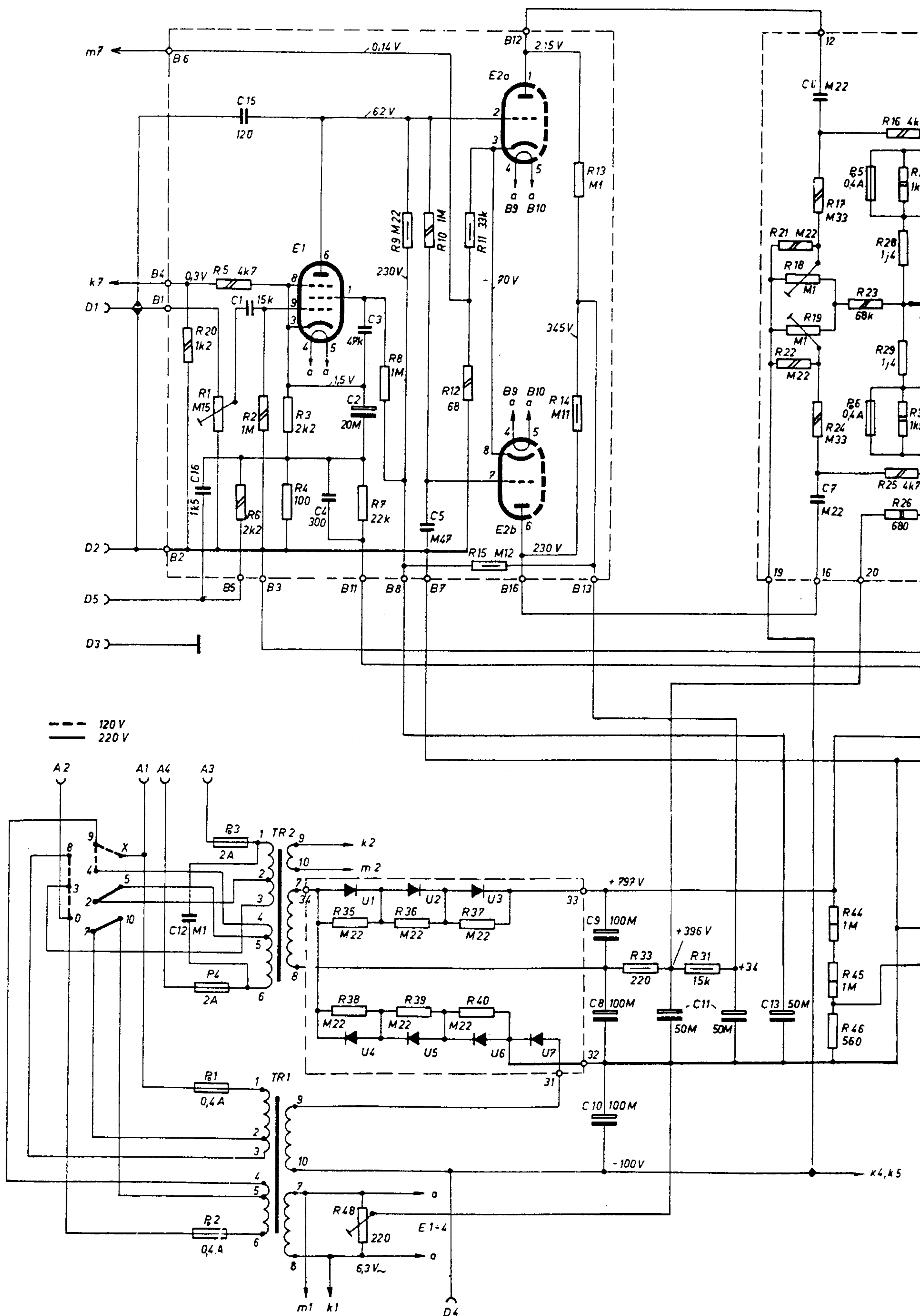
Schéma výkonového zosilňovača
